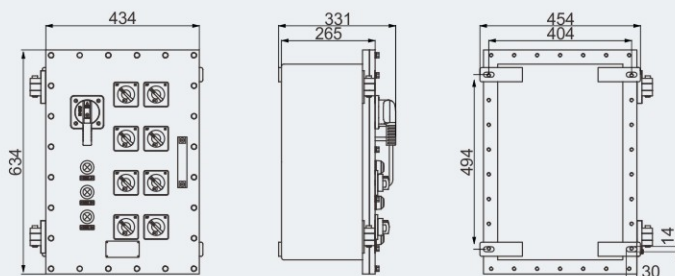
BXM(D)81-8/□/K/□
