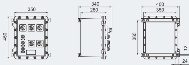
BXD81-4/□/K/□
