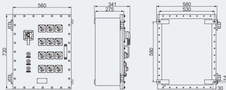
BXM(D)81-12/□/K/□
