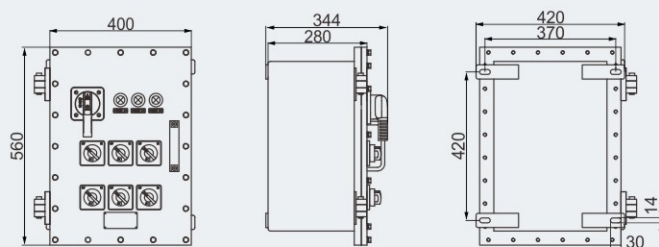
BXM(D)81-6/□/K/□
