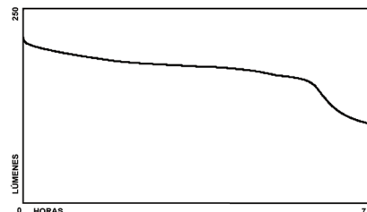
CURVA DE RENDIMIENTO XPR-5568
