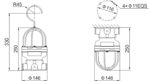
H: 手提式 Portable type
